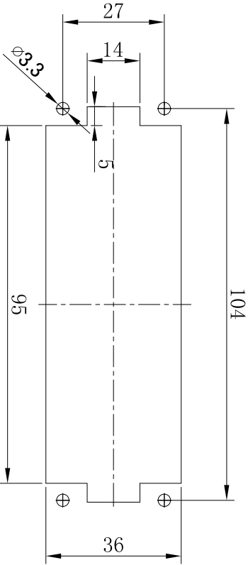
面板安装开孔图
